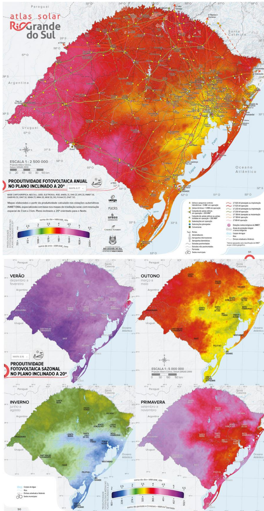
Figura 5 - Mapas do potencial fotovoltaico anual e sazonal do Estado do Rio Grande do Sul, determinado usando a metodologia apresentada neste trabalho.
