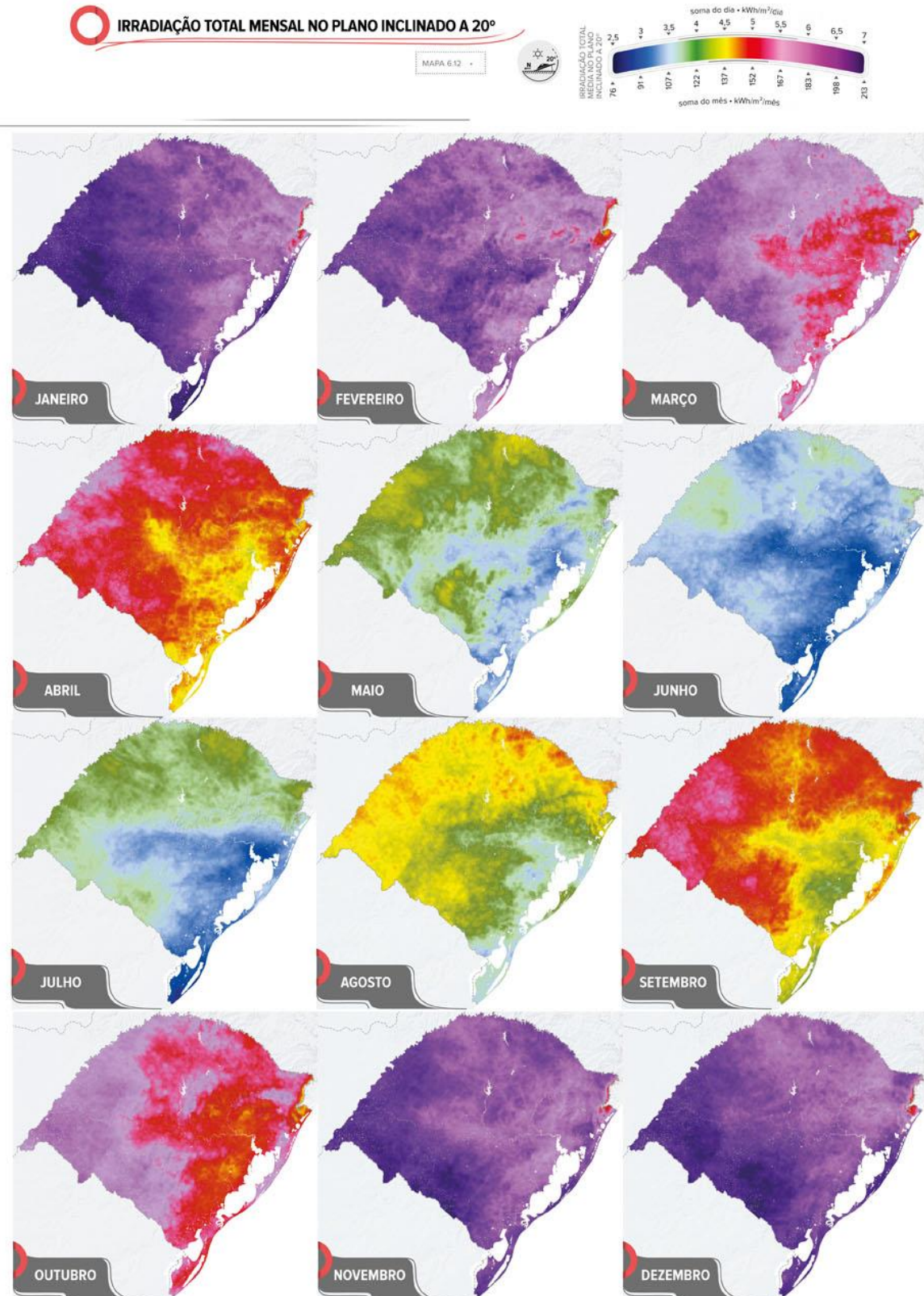
Figura 3 - Mapas de irradiação mensal para superfície inclinada de 20° voltada para Norte no RS.
